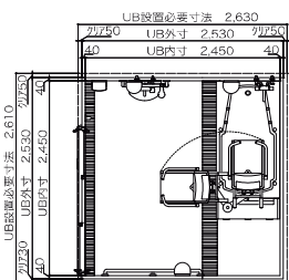
2424サイズ ※個粋プラス/チルト 浴室内寸法: 2,450×2,450mm
