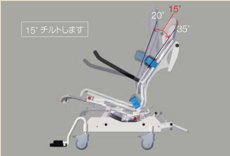
チルトチェア CC-120TA (穴あき座面) 寸法: W670×L996×H1,154(通常時) W670×L1,055×H1,085(チルト時)
