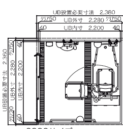
2222サイズ ※個粋プラス/コンパクト 浴室内寸法: 2,200×2,200mm
