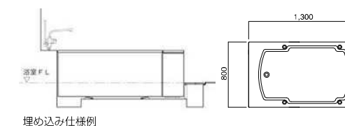
埋め込み仕様例
