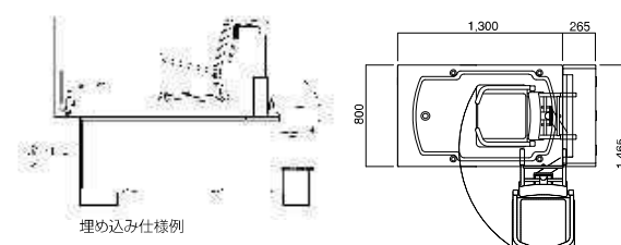
個粋コンパクト(埋め込み)
