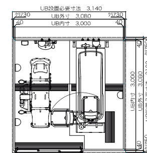
3030サイズ ※個粋コンチェルト 浴室内寸法: 3,000×3,000mm
