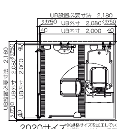
2020サイズ ※個粋コンパクトのみ設置可能。 浴室内寸法: 2,000×2,000mm
