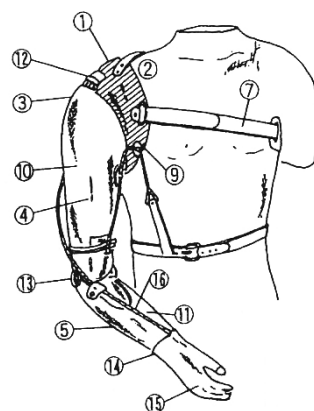
能動式（ハンド型手部付）
