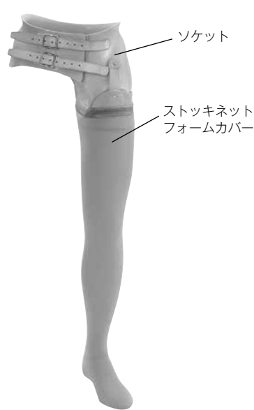
骨格構造（カナダ式）
