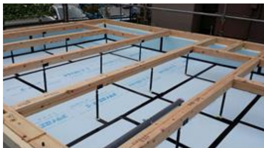
床下基礎断熱=家全体の断熱を可能にし、部屋間の温度差を解消
